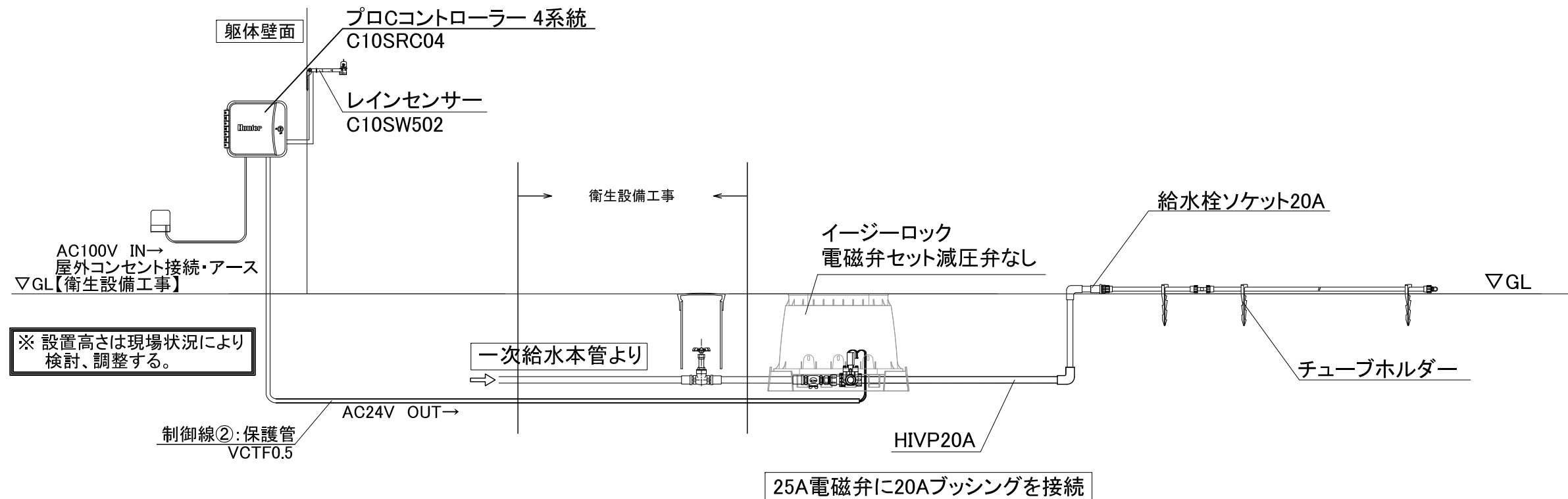
立面図
